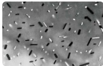
抗菌熱処理後の微視組織の一例 (黒色、白色の粒子は \epsilon -Cu相)
